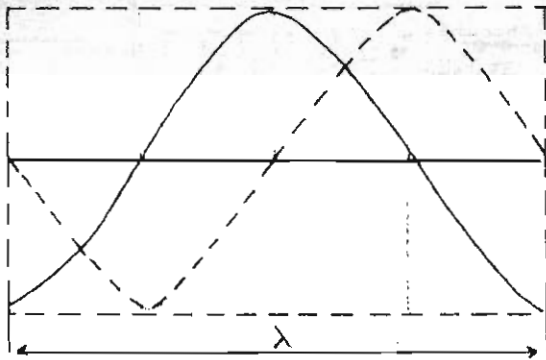
Afh. 19: De Zeppelin-antenne, waarin een hele golflengte wordt gehalveerd in een 1/2 golf straler met een twee-draads voedingslijn die 1/4 golf (of veelvoud daarvan) lang moet zijn. Alleen dan treedt er stroomvoeding op. Voor harmonischen is spanningsvoeding in het koppelpunt nodig.
