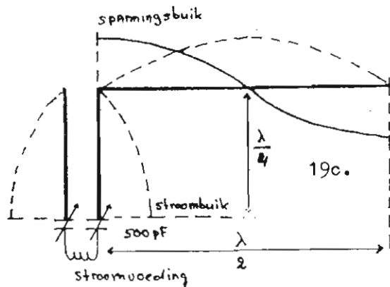
Afh. 19: De Zeppelin-antenne, waarin een hele golflengte wordt gehalveerd in een 1/2 golf straler met een twee-draads voedingslijn die 1/4 golf (of veelvoud daarvan) lang moet zijn. Alleen dan treedt er stroomvoeding op. Voor harmonischen is spanningsvoeding in het koppelpunt nodig.
