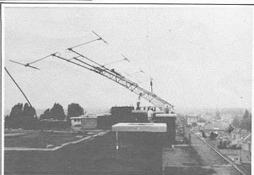
OPHIJSEN VAN DE 30 METER HOGE NIEUWE ZENDMAST
