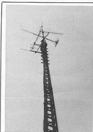
Zendmast Radio Montebaldo, waar via gerichte antennes het signaal van de (5 x) 2 kW zenders vertrekt, bovenop verschillende hergotoppen.
