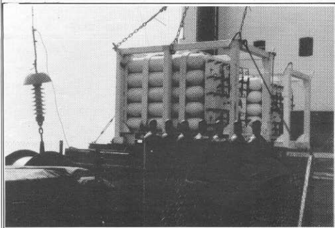
DE GASFLESSEN VOOR DE BALLOON ANTENNE BEVINDEN ZICH NOG STEEDS OP HET DEK VAN DE COMMUNICATOR.
